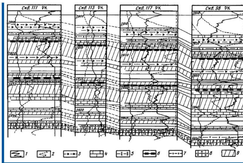
Схема сопоставления разрезов баженовской свиты по одной из разведочных линий месторождения Большой Салым:
